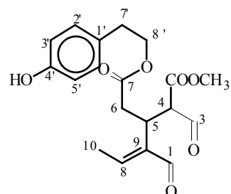
Forma dialdeidica del ligustroside aglicone
