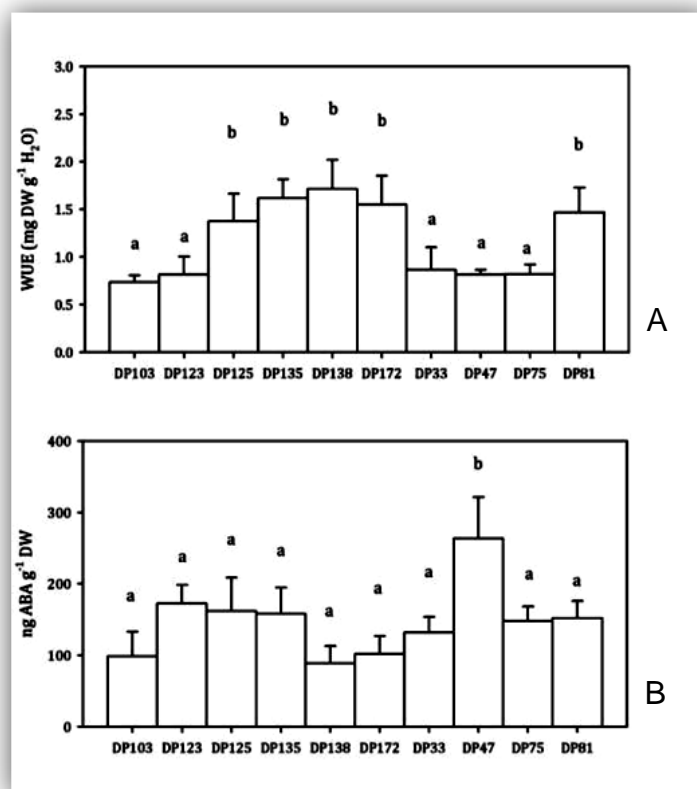
Figura 2.2. (A). Distribuzione fenotipica relativa alle 5 accessioni con bassi valori di WUE (a) e valori elevati di WUE (b). I dati riportati fanno riferimento alle medie delle accessioni in tutte e sei le repliche. (B). Per le medesime accessioni sono riportate le distribuzioni medie della concentrazione di ABA nelle 6 repliche.
