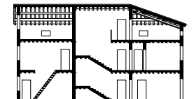
Sezione LONG A-A Sc. 1:200
