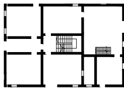
Piano TERRA Sc. 1:200
