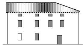
Prospetto OVEST Sc. 1:200
