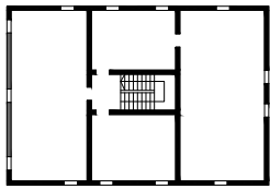
SECONDO piano Sc. 1:200
