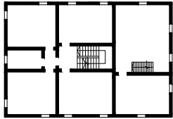
PRIMO piano Sc. 1:200
